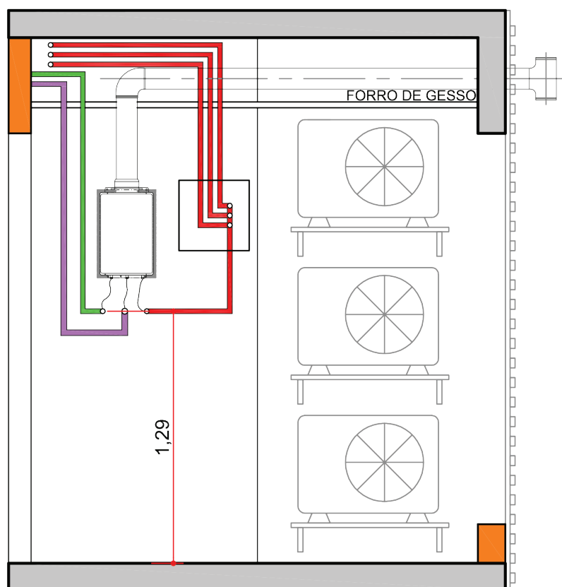
ELEVAÇÃO - 06
