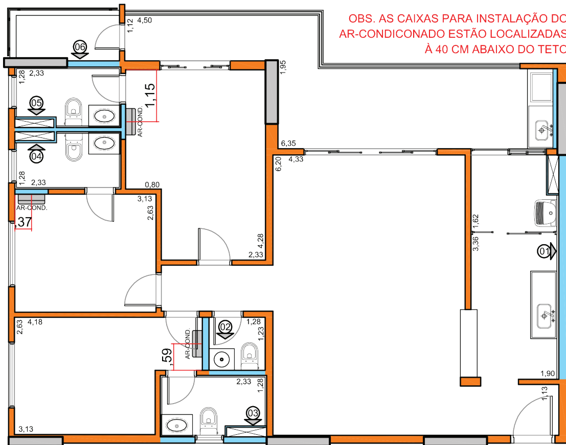
PLANTA
