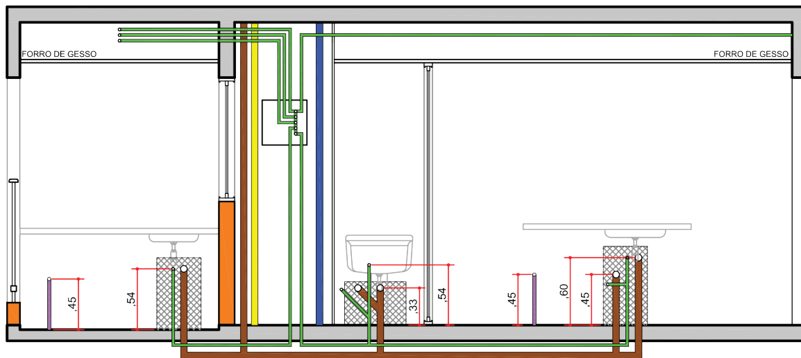
ELEVAÇÃO - 01
