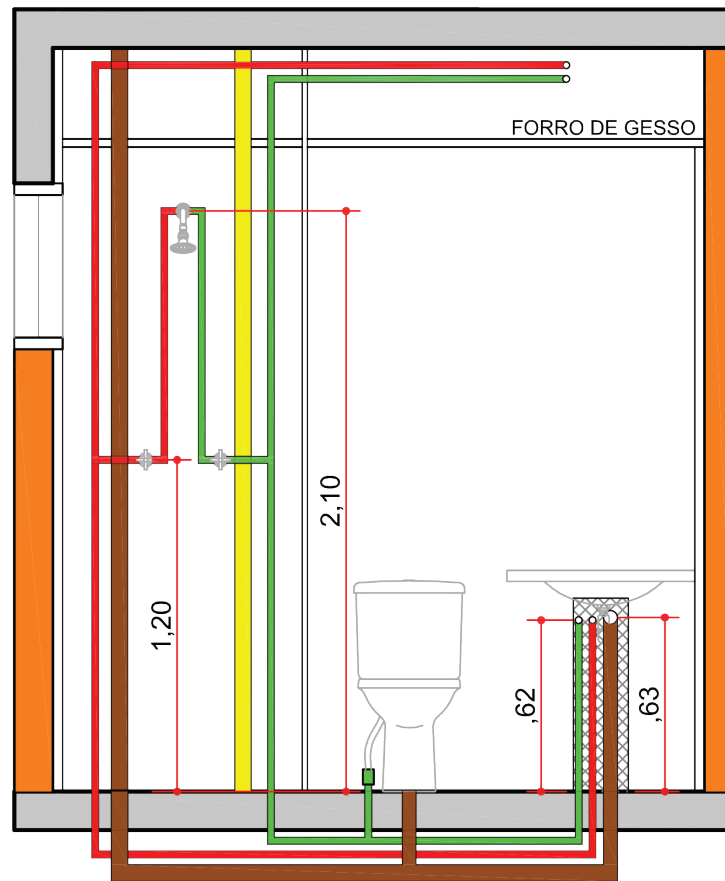
ELEVAÇÃO - 04
