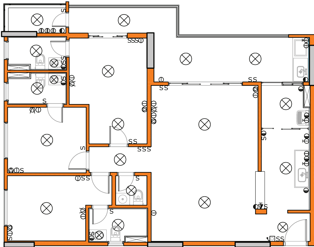
PLANTA - ELÉTRICA
