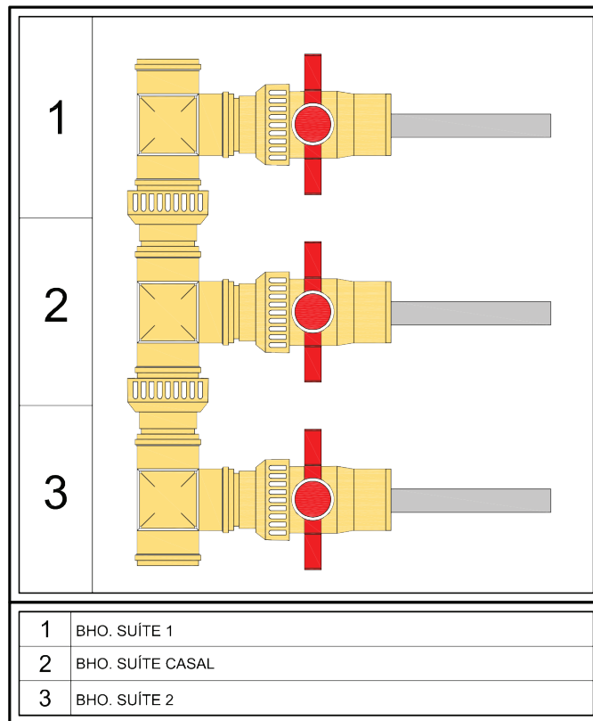
MANIFOLD ÁGUA QUENTE - ÁREA TÉCNICA
