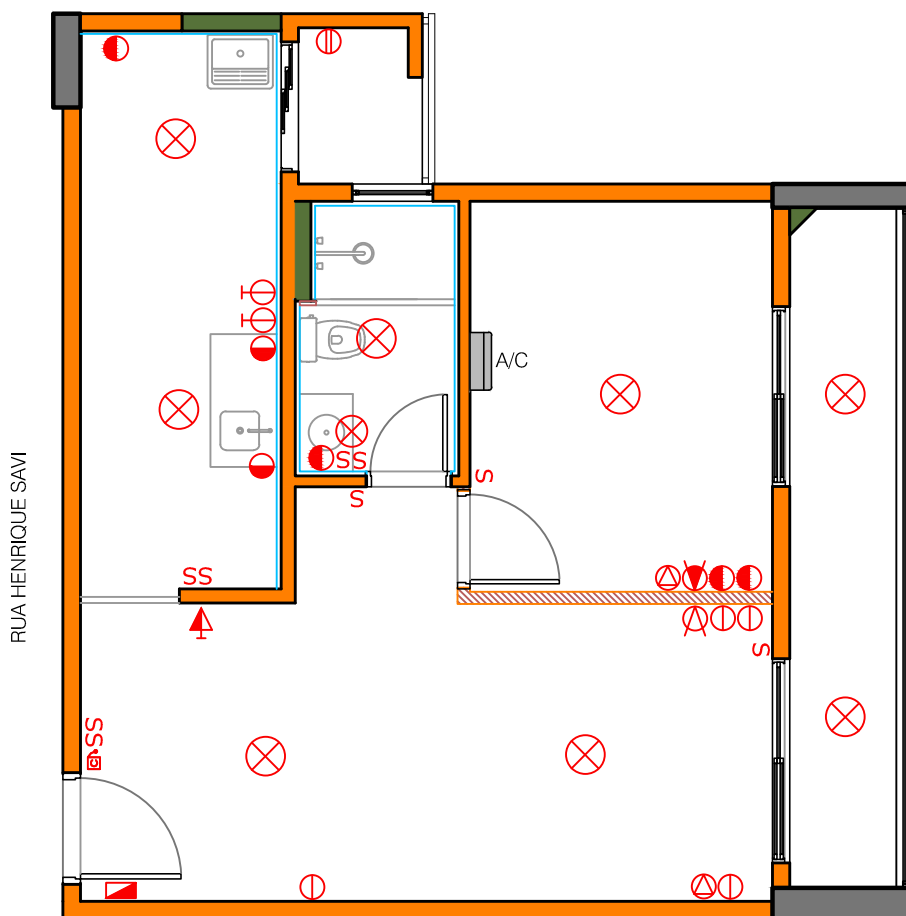
PLANTA - FINAL 04, 06, 10 E 12 SEM ESCALA
