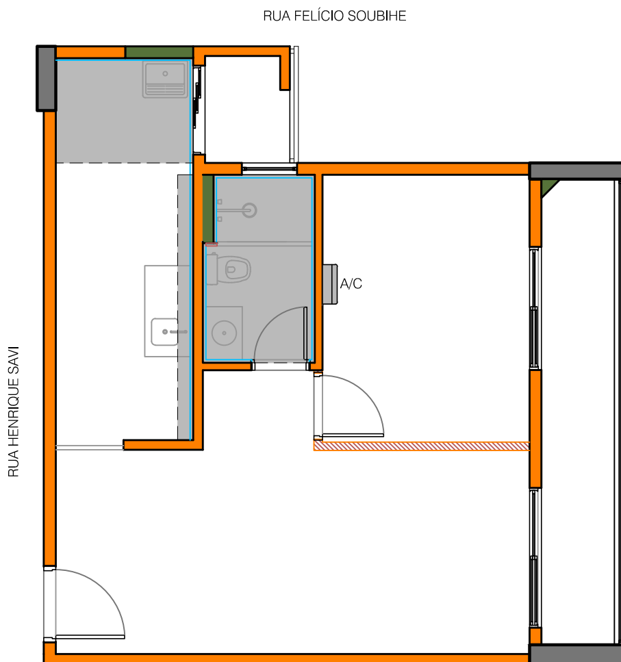
PLANTA - FINAL 04, 06, 10 E 12
