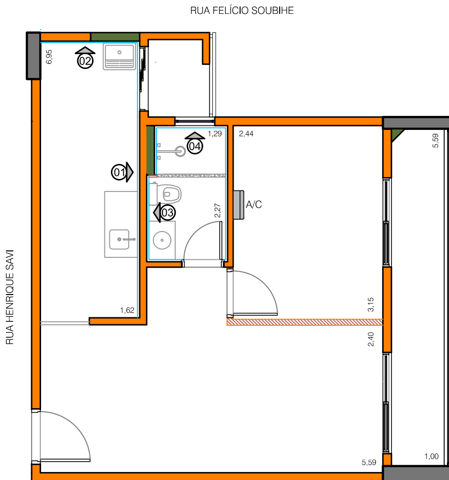
PLANTA - FINAL 04, 06, 10 E 12 SEM ESCALA
