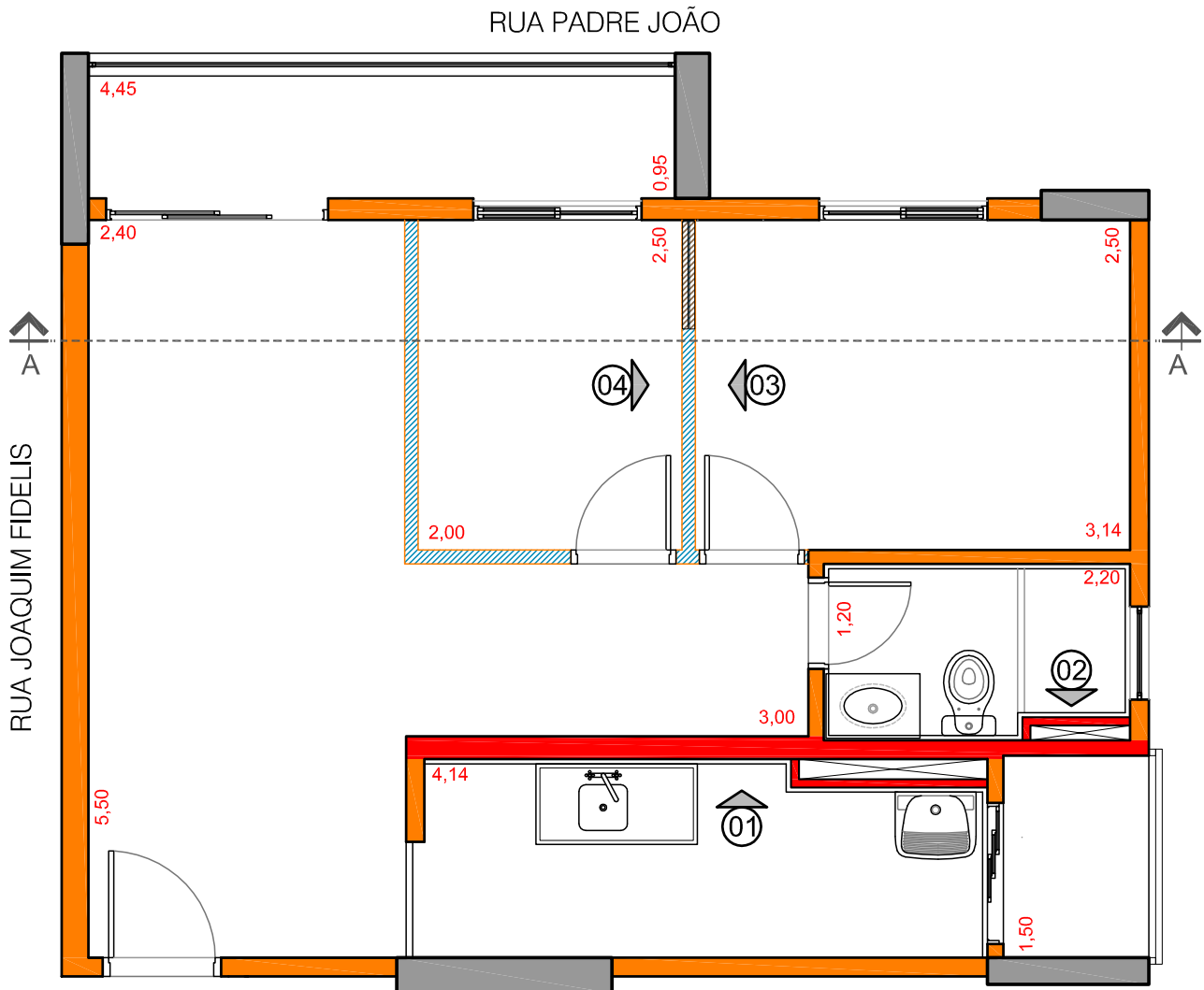
PLANTA ESCALA: 1:50
