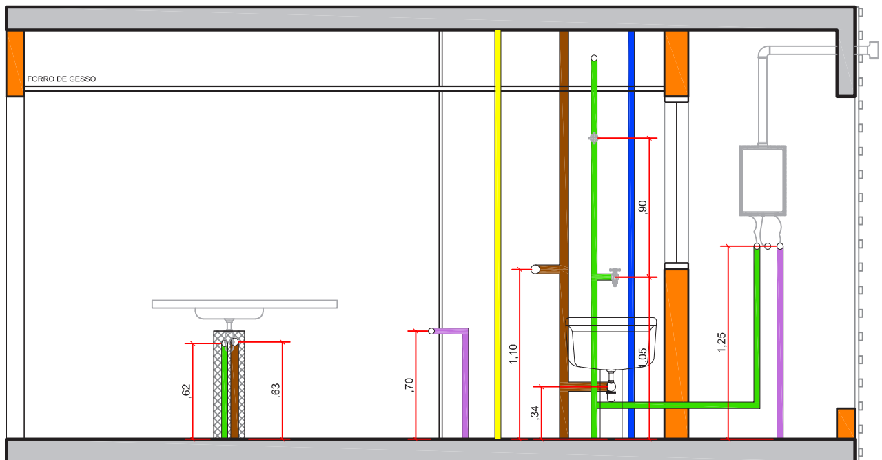
ELEVAÇÃO 01
