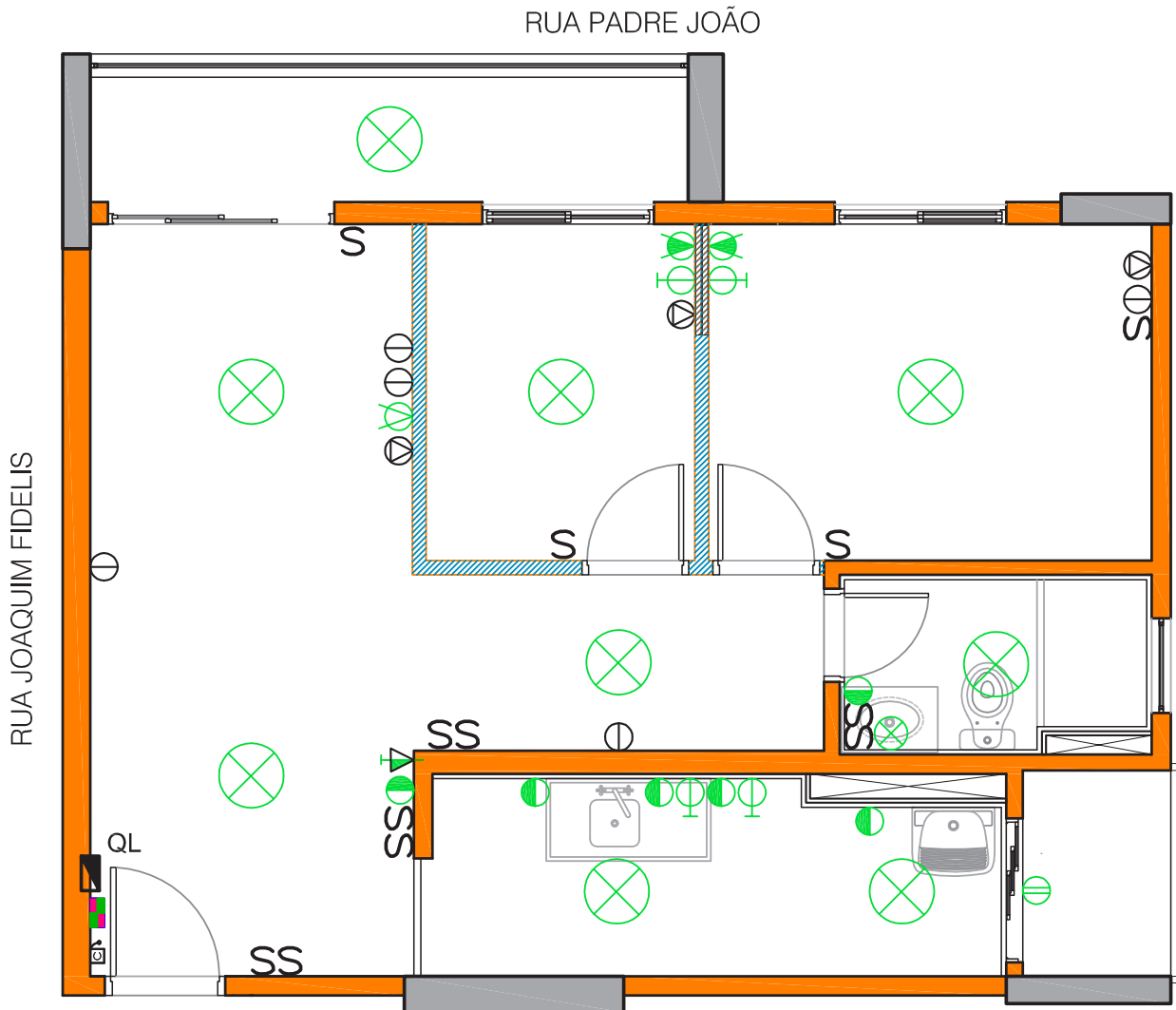
PLANTA ESCALA: 1:50
