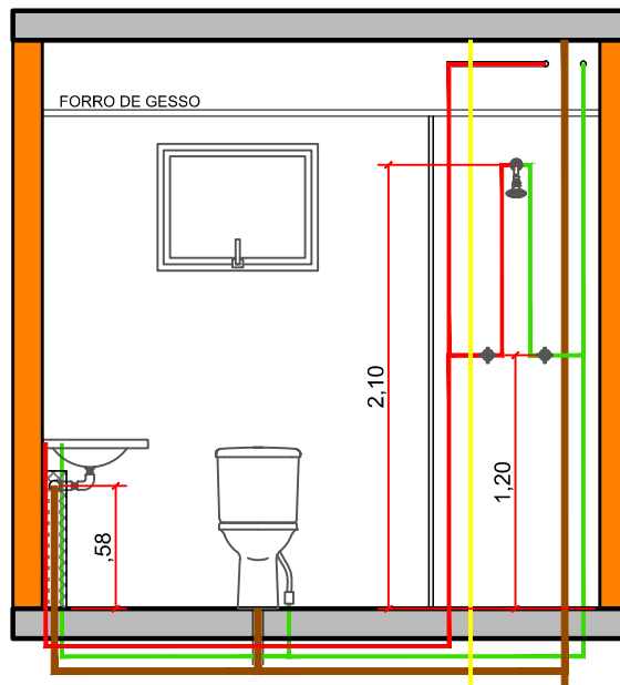
ELEVAÇÃO 05
