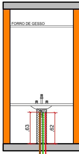
ELEVAÇÃO 06
