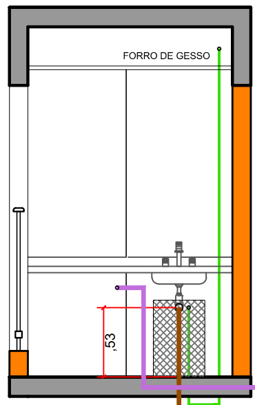
ELEVÇÃO 02
