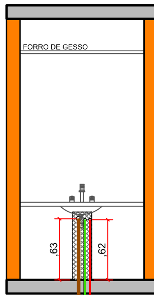
ELEVAÇÃO 04
