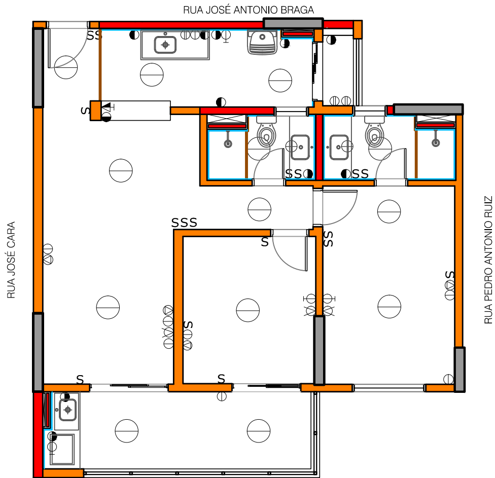
PLANTA - FINAL 04 SEM ESCALA
