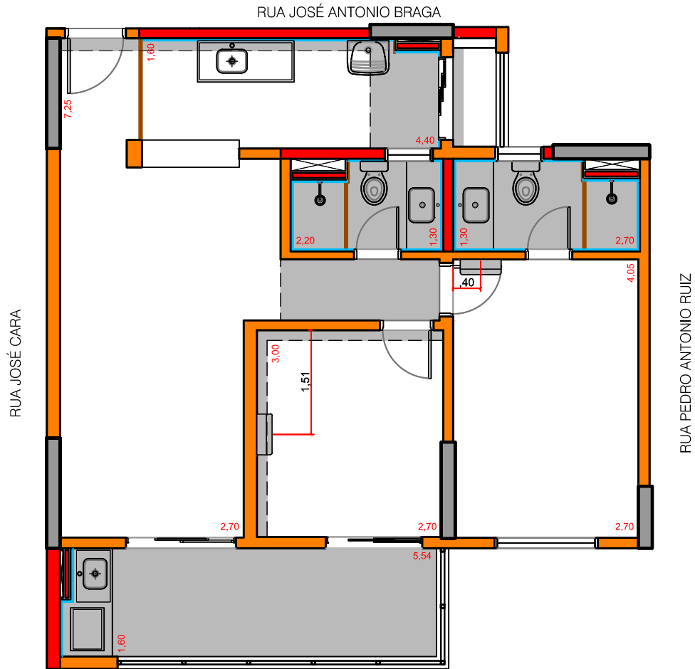
PLANTA - FINAL 04
