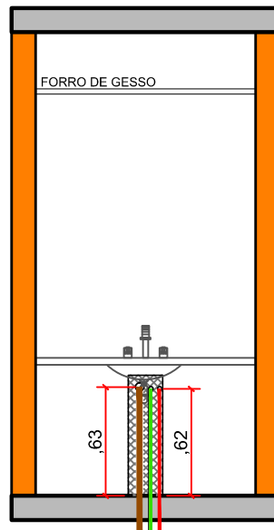
ELEVAÇÃO 04
