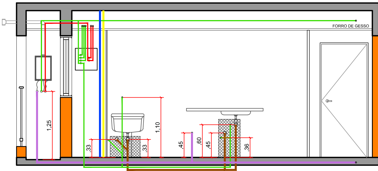
ELEVAÇÃO 01
