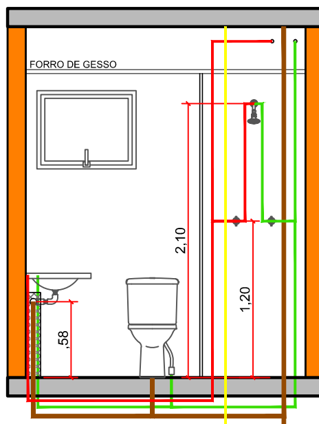
ELEVAÇÃO 03
