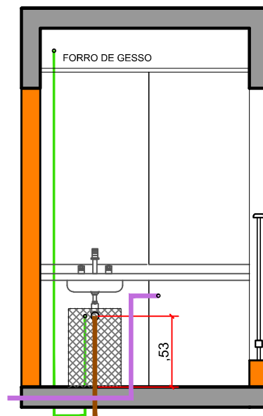
ELEVAÇÃO 02
