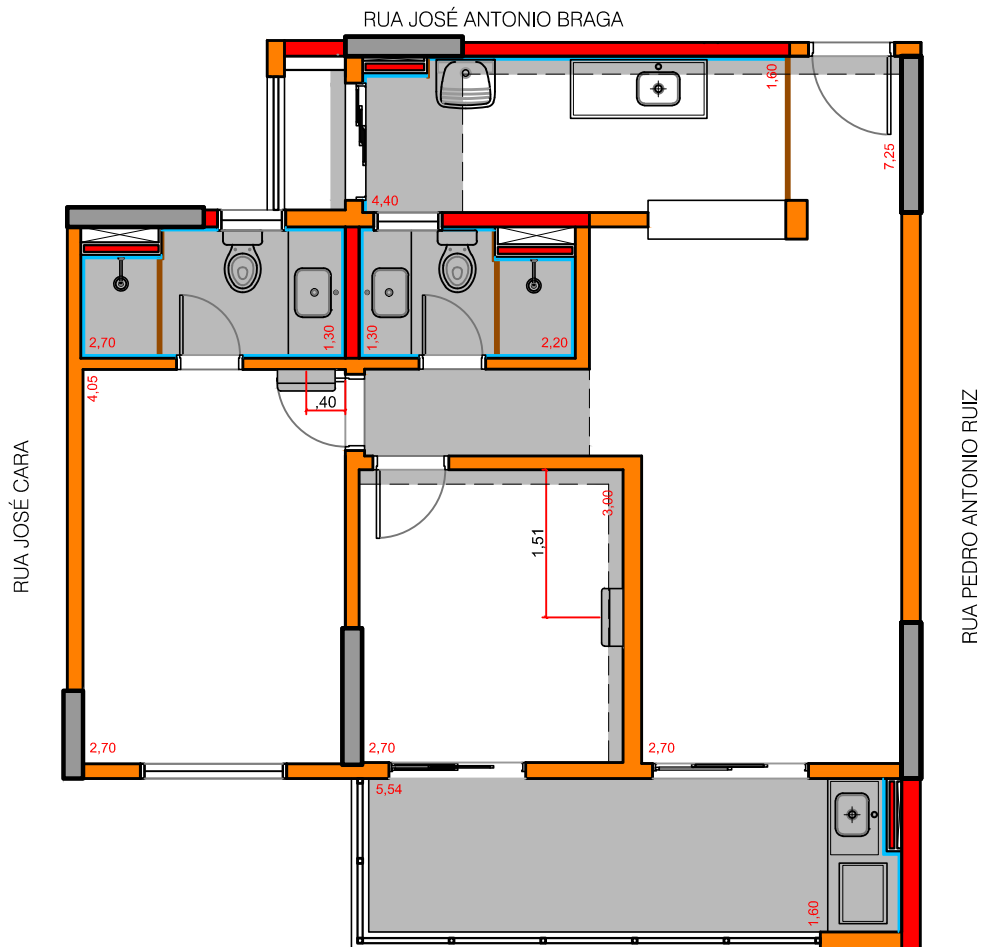
PLANTA - FINAL 03 SEM ESCALA
