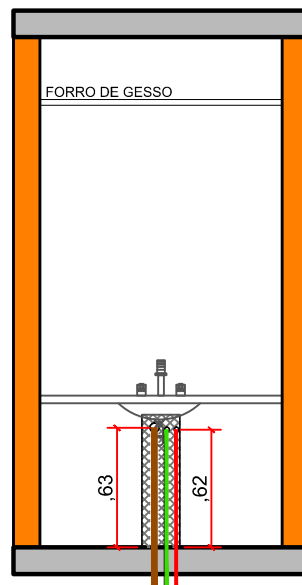
ELEVAÇÃO 06
