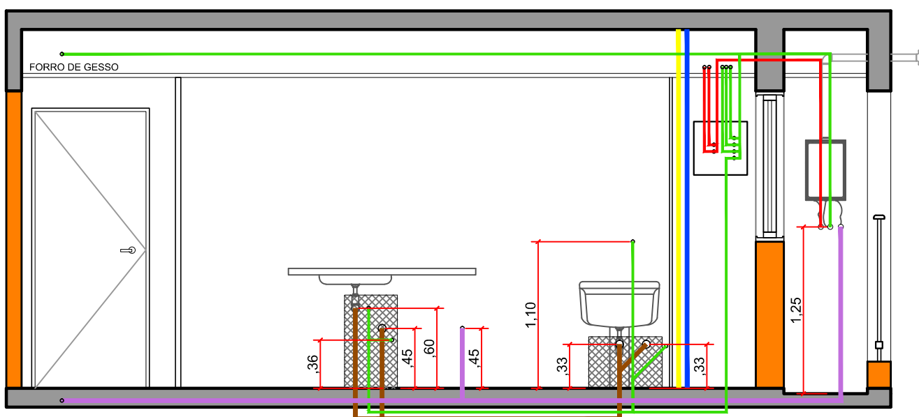
ELEVAÇÃO 01
