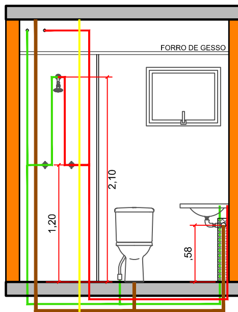
ELEVAÇÃO 03
