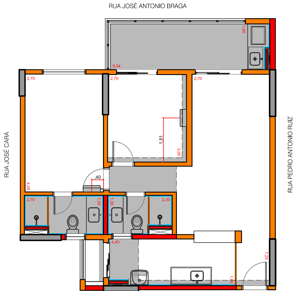
PLANTA - FINAL 02 SEM ESCALA
