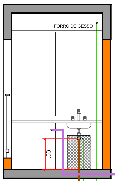
ELEVAÇÃO 02
