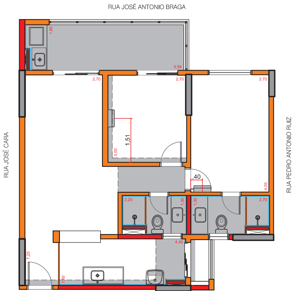
PLANTA - FINAL 01 SEM ESCALA
