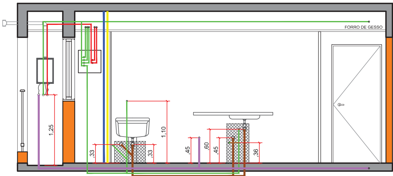
ELEVAÇÃO 01
