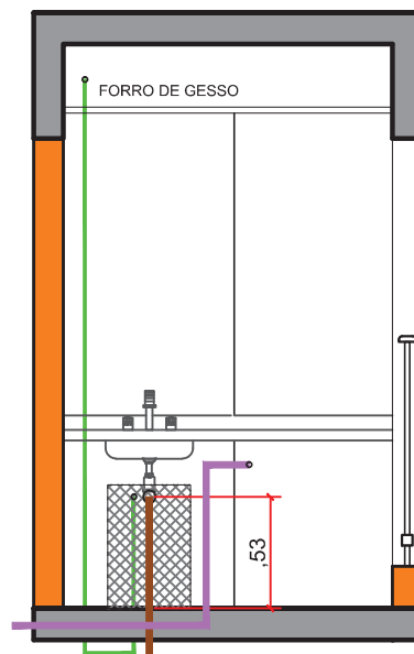
ELEVAÇÃO 02
