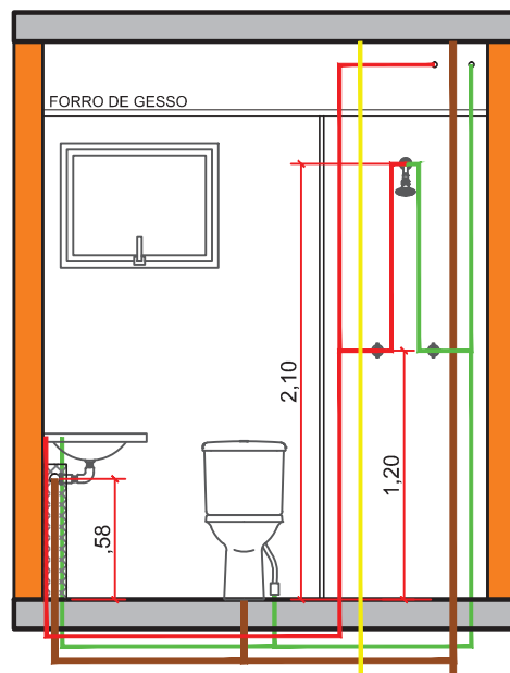
ELEVAÇÃO 03 SEM ESCALA
