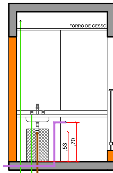
ELEVAÇÃO 03
