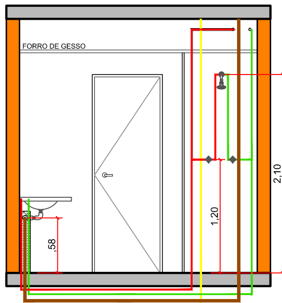
ELEVAÇÃO 06
