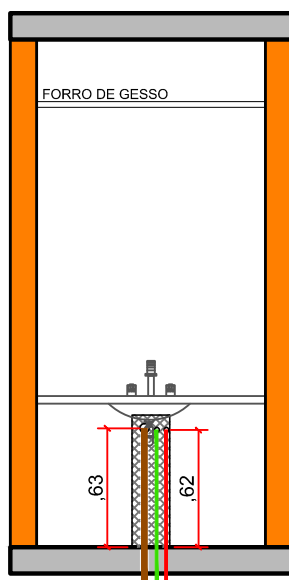
ELEVAÇÃO 04
