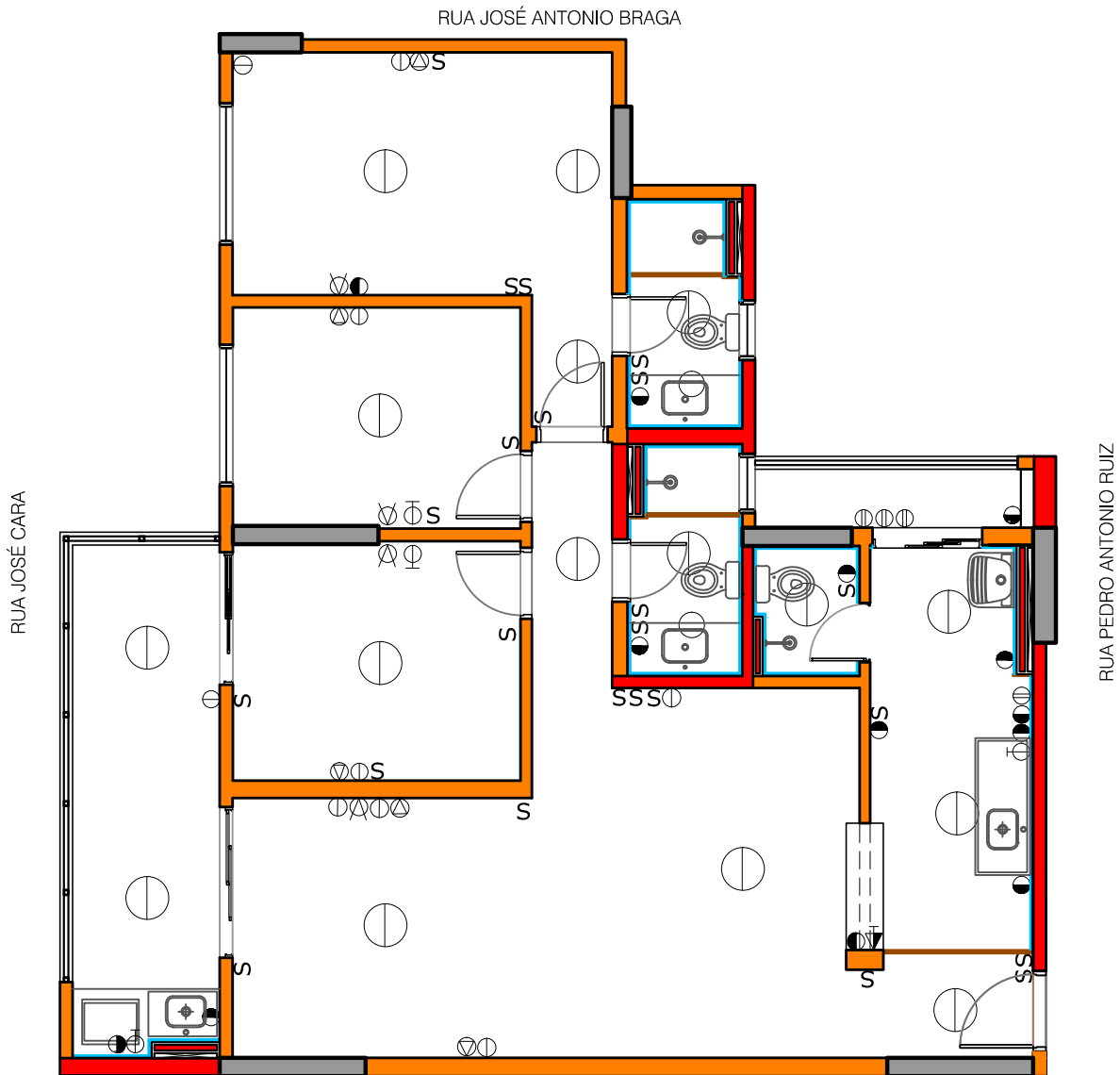
PLANTA - FINAL 01 SEM ESCALA
