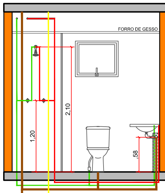
ELEVAÇÃO 08
