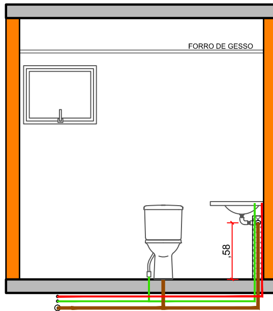
ELEVAÇÃO 05 SEM ESCALA
