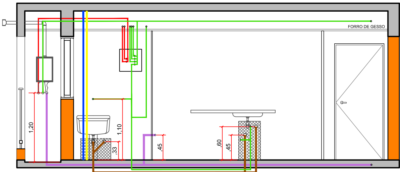
ELEVAÇÃO 01
