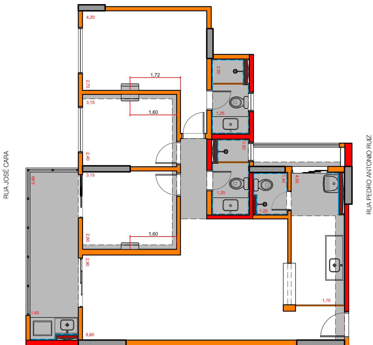
PLANTA - FINAL 01
