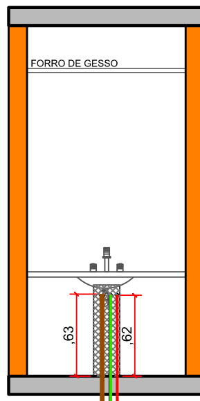
ELEVAÇÃO 07
