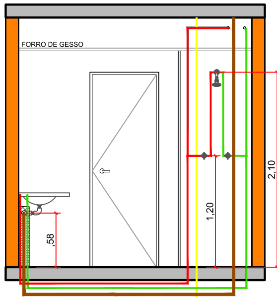
ELEVAÇÃO 06
