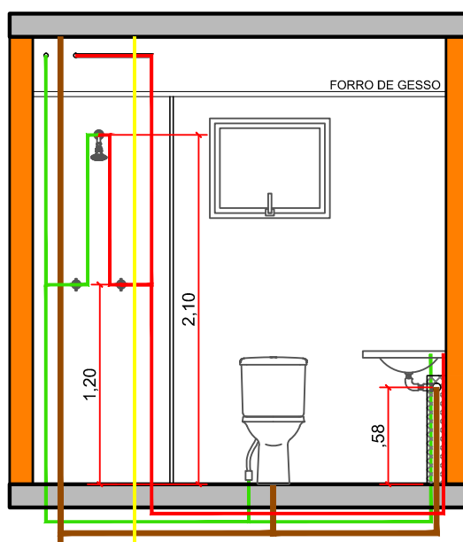
ELEVAÇÃO 08
