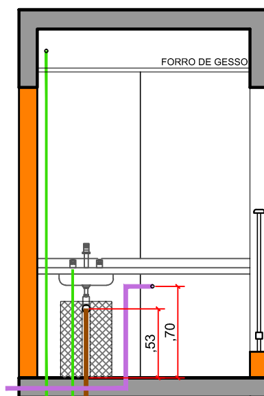
ELEVAÇÃO 03
