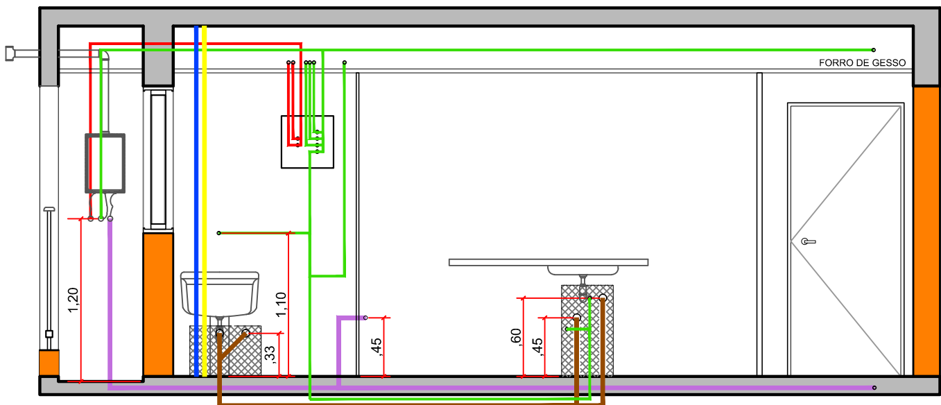
ELEVAÇÃO 01
