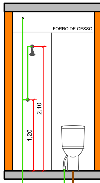
ELEVAÇÃO 02
