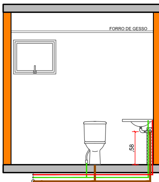
ELEVAÇÃO 05
