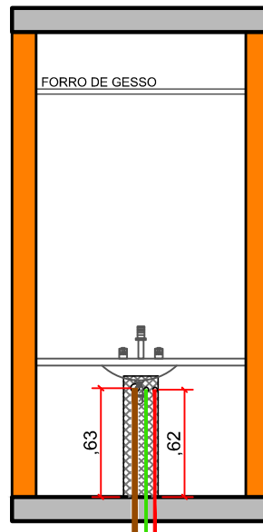
ELEVAÇÃO 04
