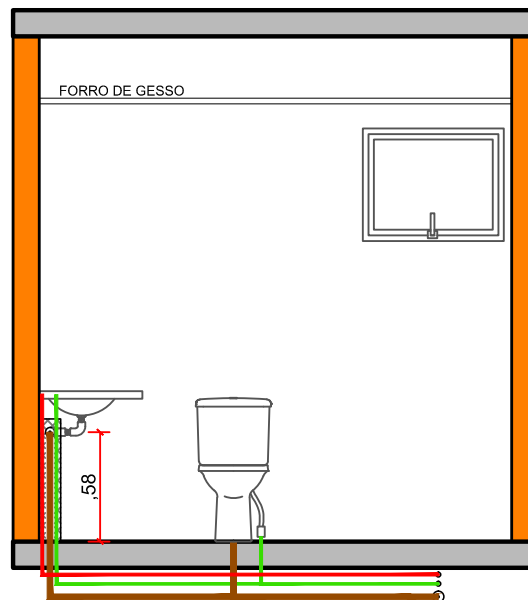
ELEVAÇÃO 05
