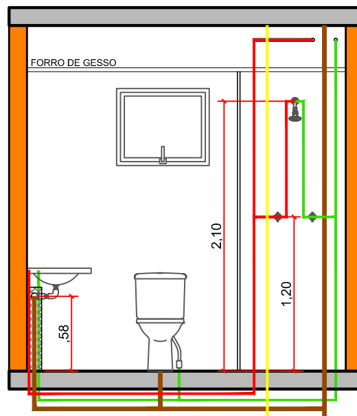
ELEVAÇÃO 08
