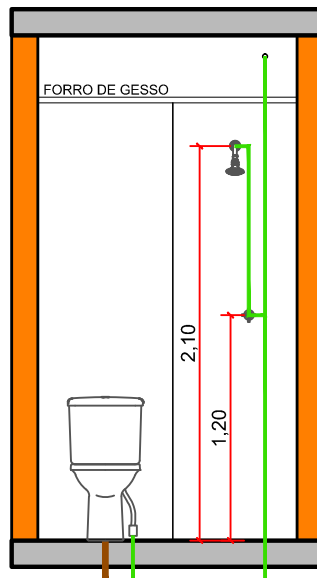
ELEVAÇÃO 02
