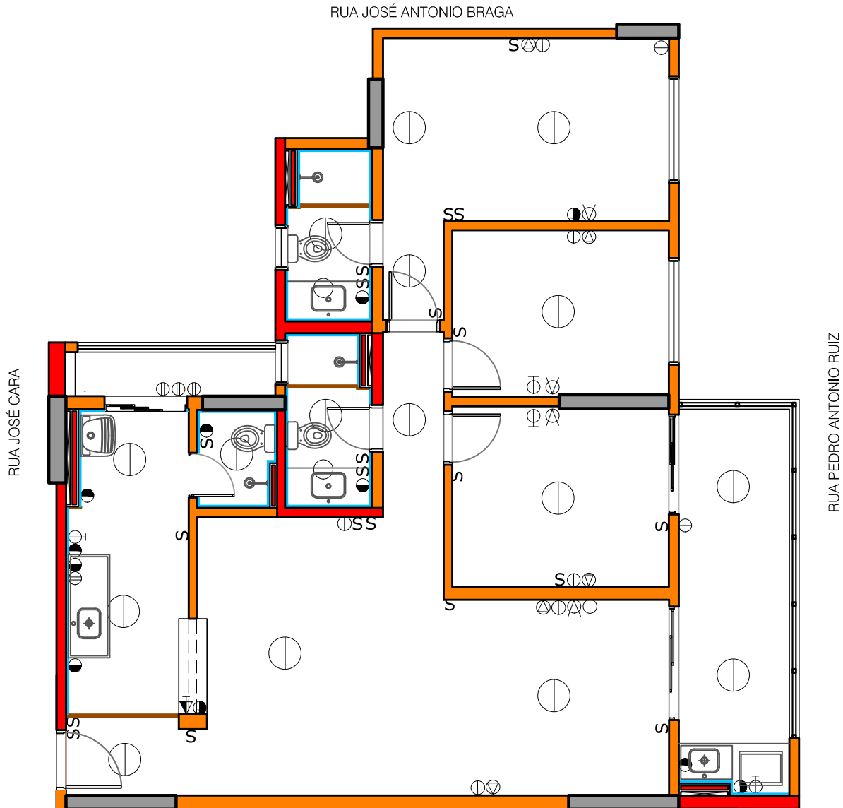
PLANTA - FINAL 04 SEM ESCALA
