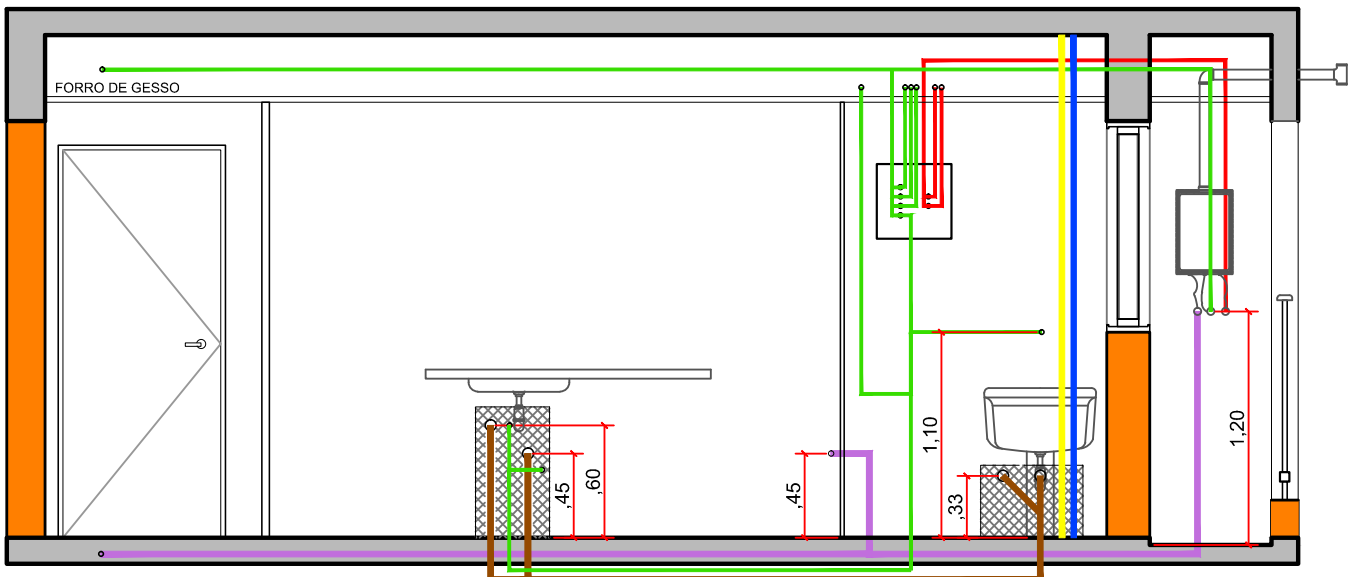
ELEVAÇÃO 01
