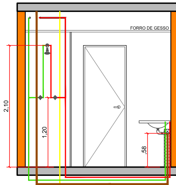
ELEVAÇÃO 06
