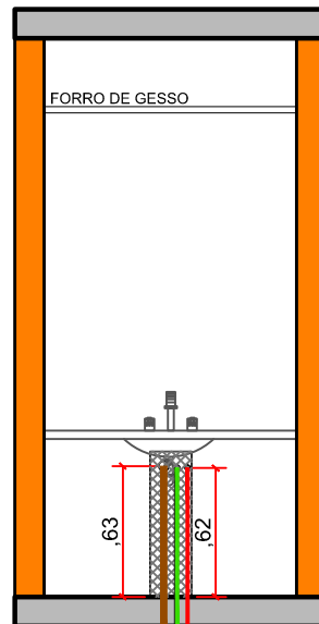
ELEVAÇÃO 07
